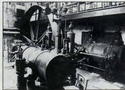
De stoommachine van het Nationaal Museum van de Speelkaart, toestand 1978.
