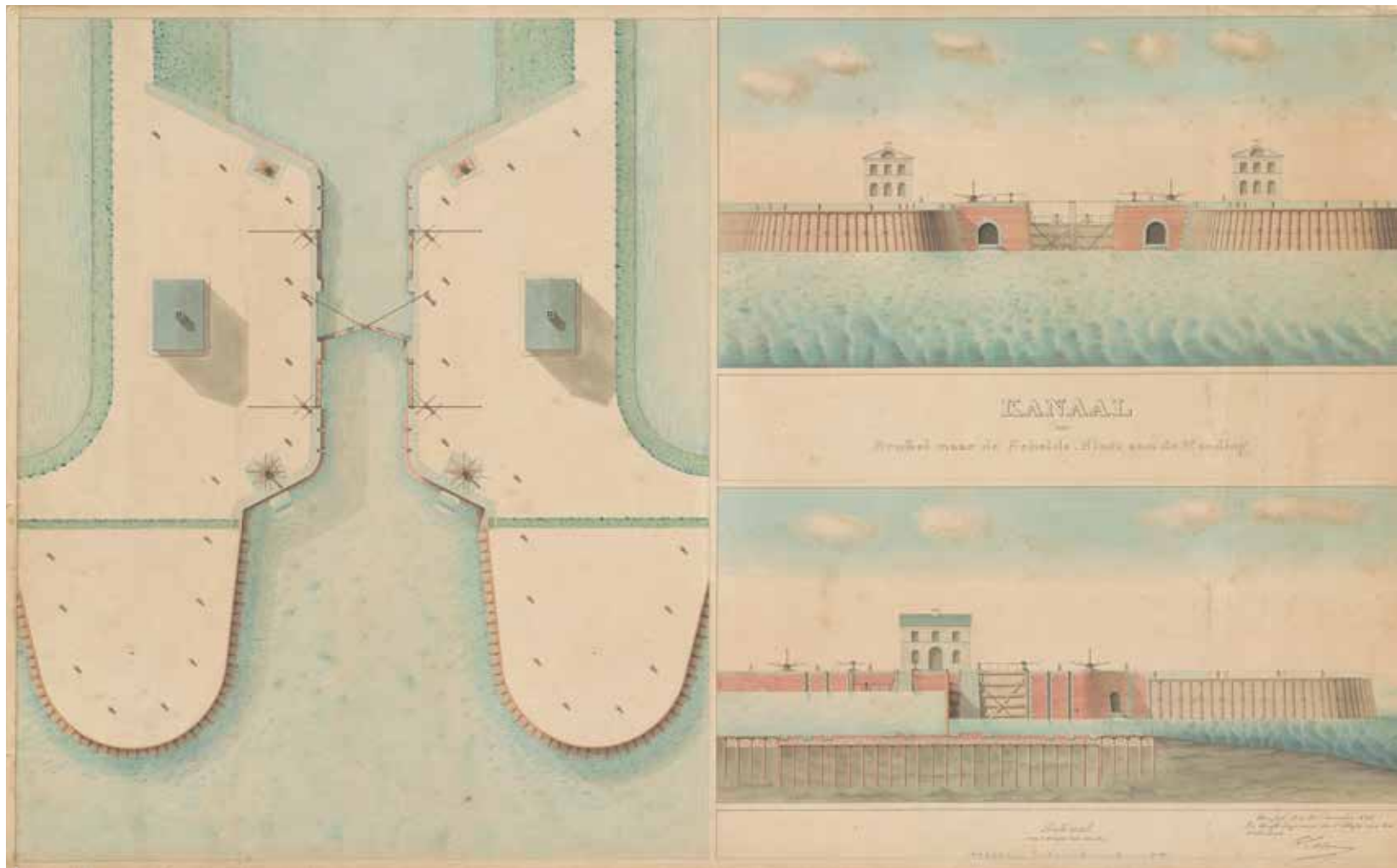
Plan van de sluis in Klein-Willebroek op het kanaal Brussel-Schelde 1825 NATIONAAL ARCHIEF DEN HAAG
